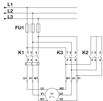
Fig. 11 Ligações estrela triângulo
