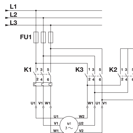
Fig. 11 Conexiuni stea-triunghiulară
