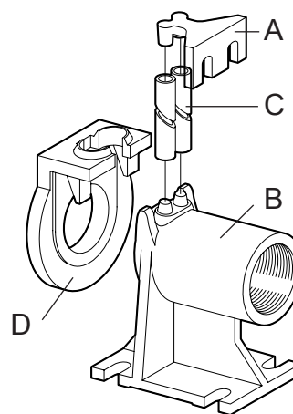
Fig. 7 Piede d'accoppiamento
