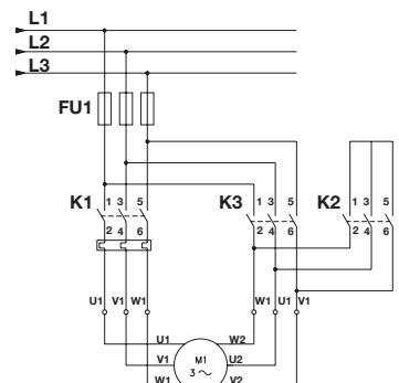
Afb. 11 Ster-driehoekaansluitingen
