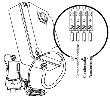
Afb. 9 Schakelpaneel voor laagspanningspompen
