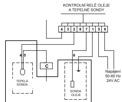
C= DÁLKOVÝ OVLADAČ ČERPADLA 4-5-6 = ČÍSLOVÁNÍ VODIČŮ KABELU
